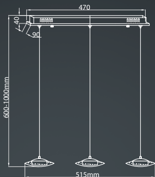
ML 413 15W [79W] 1050 lm
