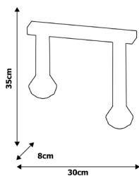
MLP 3871 2xE27 60W
