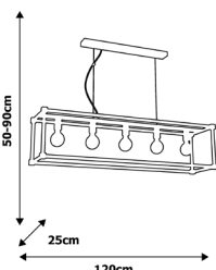
MLP 3730 5xE27 60W
