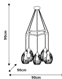
MLP 4738 5xE27 60W
