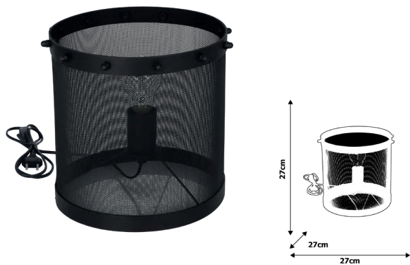
MLP 3717 1xE27 60W
