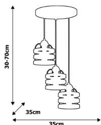
MLP 787 3xE27 60W
