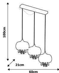
ML 3846 3xE14 40W
