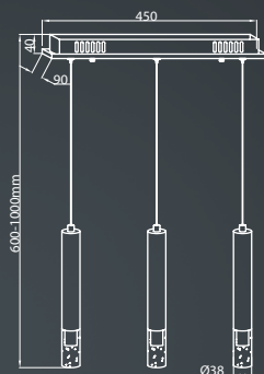
ML 189 15W [79W] 1050 lm
