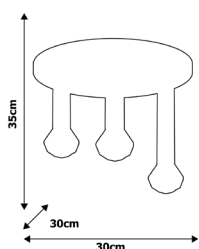
MLP 3870 3xE27 60W
