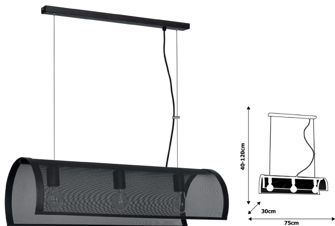
MLP 4404 3xE27 60W
