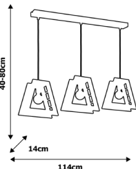
MLP 3749 3xE27 60W
