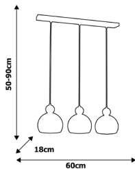
MLP 4245 3xE27 60W
