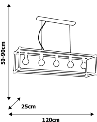
MLP 3767 5xE27 60W
