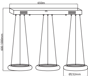
ML 420 36W [179W] 2520 lm
