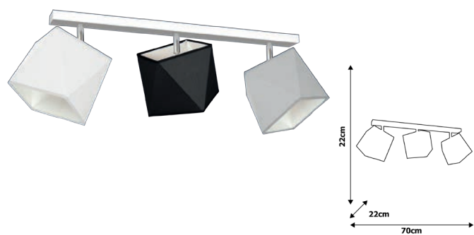
MLP 4708 3xE27 60W
