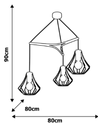
MLP 4194 3xE27 60W
