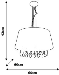
MLP 3706 5xE14 40W
