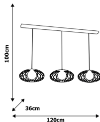
MLP 4424 3xE27 60W
