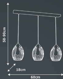
MLP 4732 3xE27 60W
