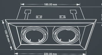
● 473 ● 475 GU10, 14W (74W), 1120 Lm
